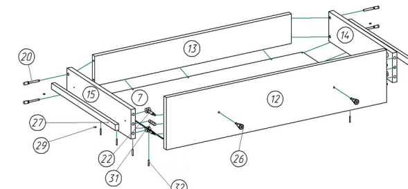
Рис.6 Сборка ящиков
